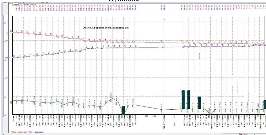
Пьезометрический график от котельной Больничного городка до дома № 6 по ул. Вавилина
