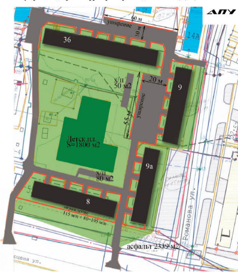
Благоустройство дворовой территории в районе домов №№10, 9, 9а, 8 м-она Гоголя
